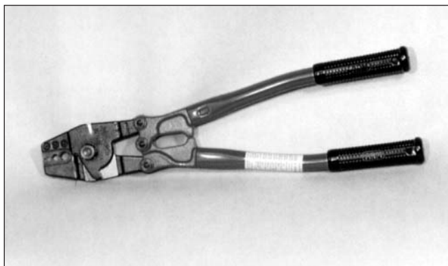
Univerzální kleště HSC 350 pro svorky od OS-1A do OS-3B
