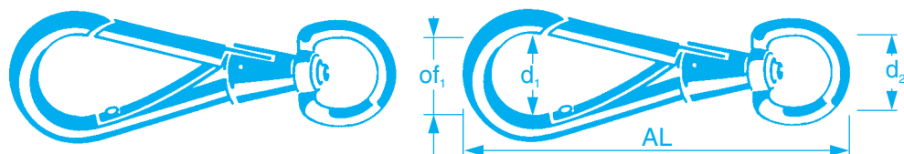
Kleštinové karabiny
