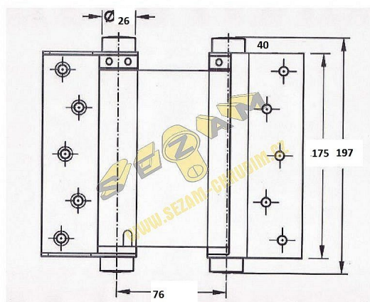
rozměr pro pant velikosti 175
