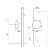
vnější štít
