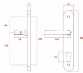
vnitřní štít
