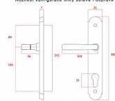
vnitřní štít
