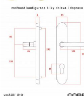
možnost konfigurace kliky doleva i doprava vnější štít COBRA
