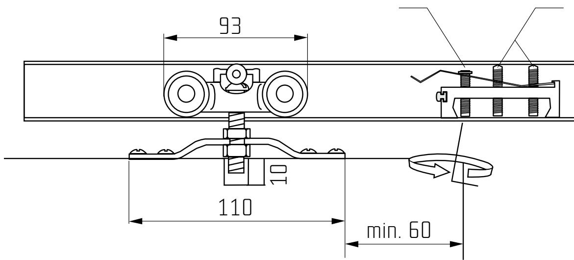
seřízení přitlaku brzdy
